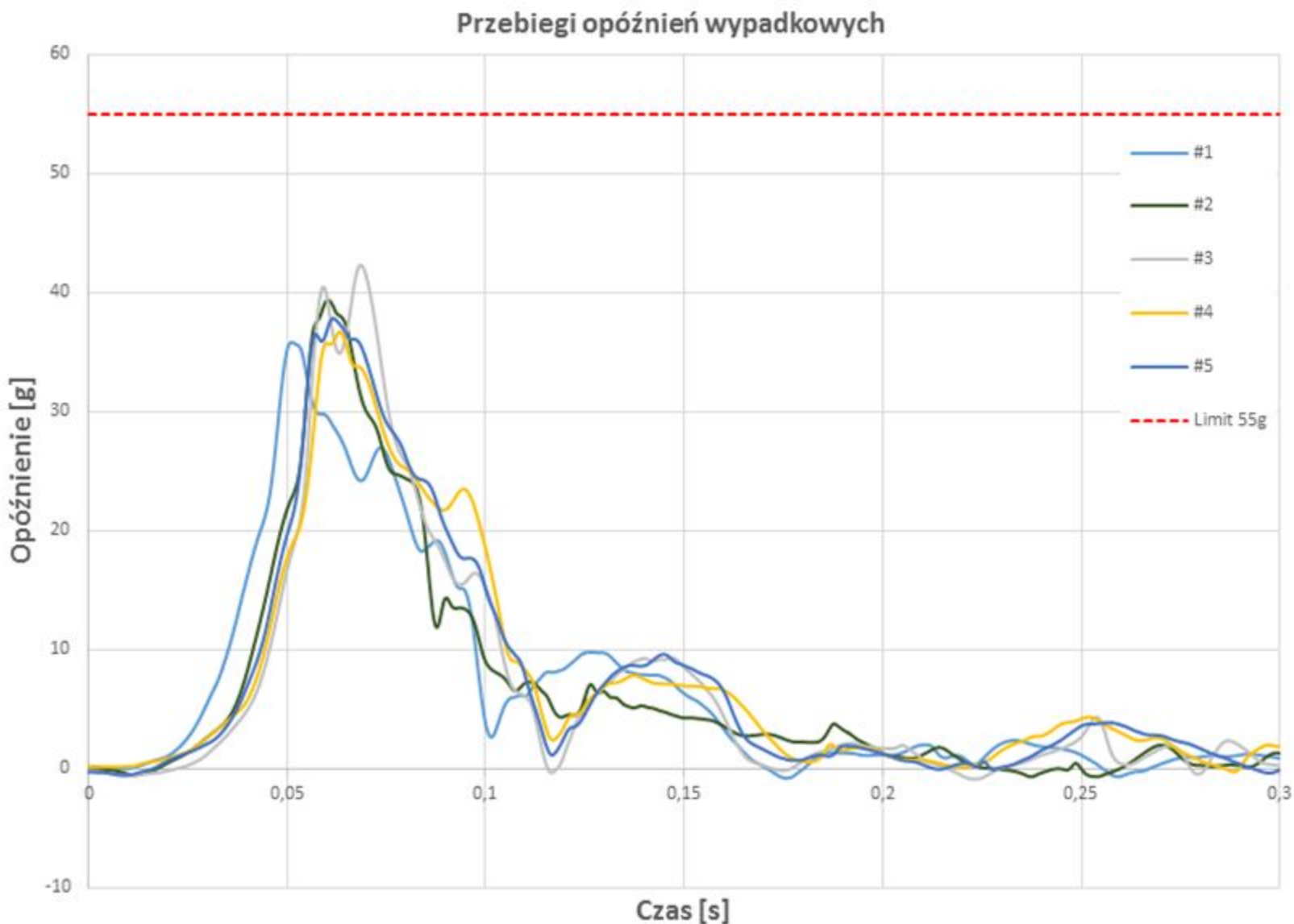
Wykres 7. Przebiegi opóźnienia wypadkowego torsu manekina 32 kg podczas testów dynamicznych Graph 7. Decelerations of the chest for 32 kg dummy during dynamic tests
